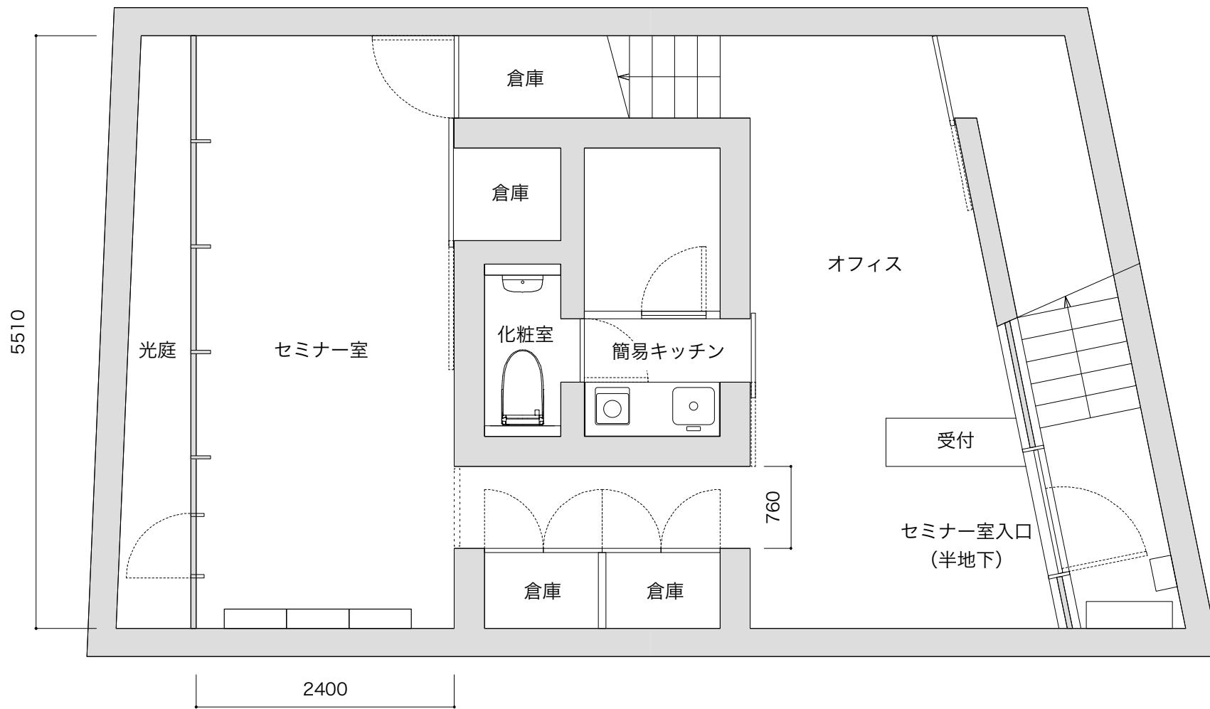
地下1階平面図 S=1:50
